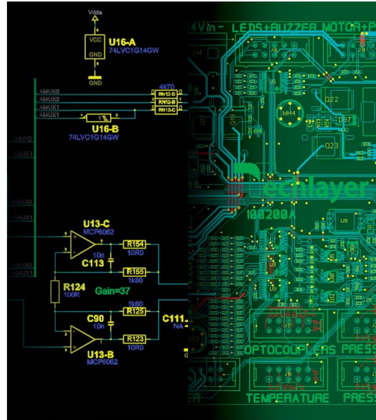
Schema ontwerp
